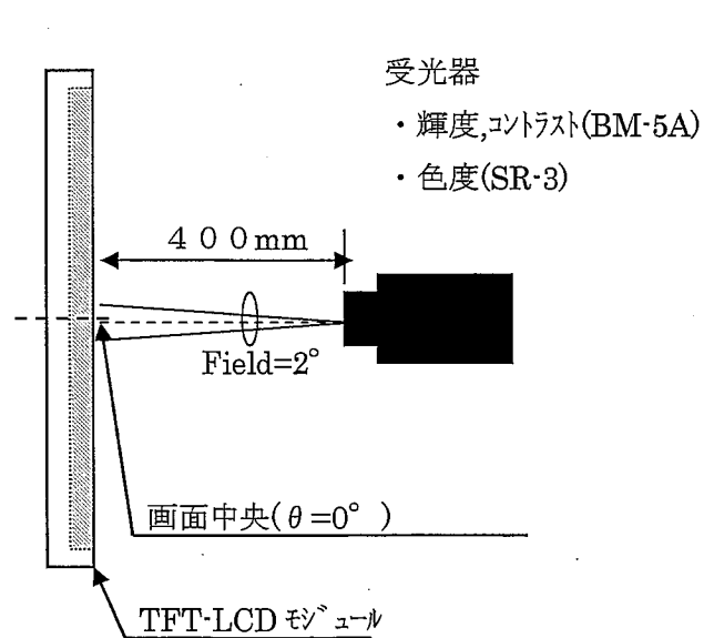
図 2-2 輝度/コントラスト/色度特性測定方法
