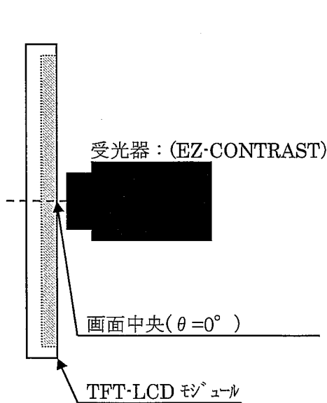
図 2-1 視野角特性/応答速度測定方法
